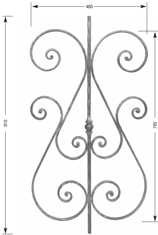
MARTELÉ ART. PAN21-14-910 H. 910 - □14 - Vol. □14x8
