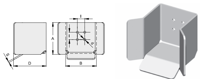
ART. 2031 A 130 B 125 D 133 I 30 d 9 S 5
