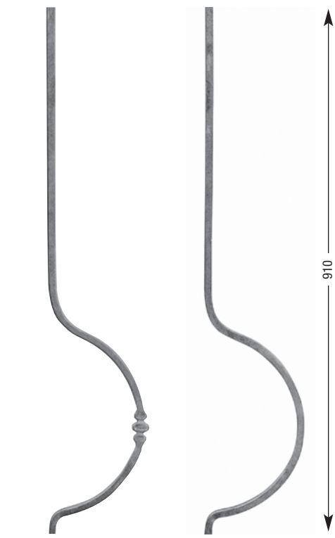
LISSE ART. 103GLS-14-910 H. 910 - □14
