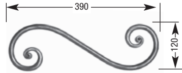
LISSE ART. VR6-14 Ø 14
