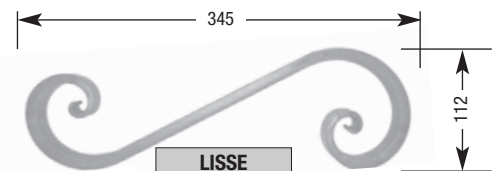
LISSE ART. V403L □ 20x10
