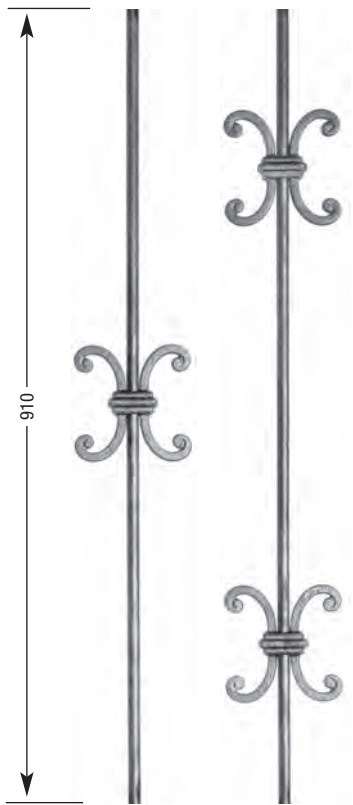
ART GV1 - Trou Ø 14 H 130 - L 130
