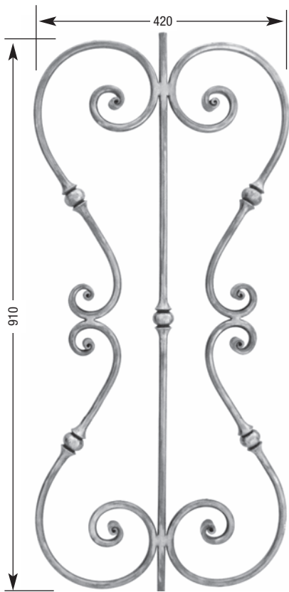
LISSE ART. PAN15L-14-910 H. 910 - Ø14
