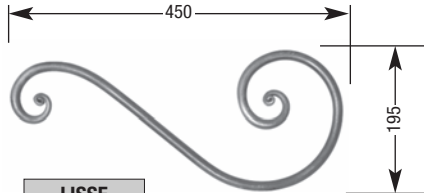
LISSE ART. VR5-14 Ø 14
