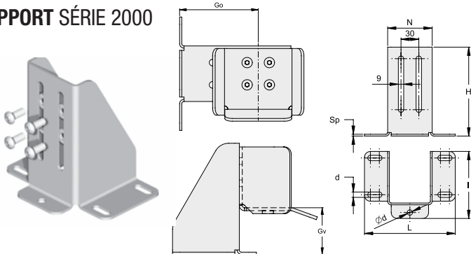
SUPPORT POUR BATTANT FIXATION MURALE OU AU SOL ART. 1035 A 210 B 150 D 177 I 92 d 5 S 11
