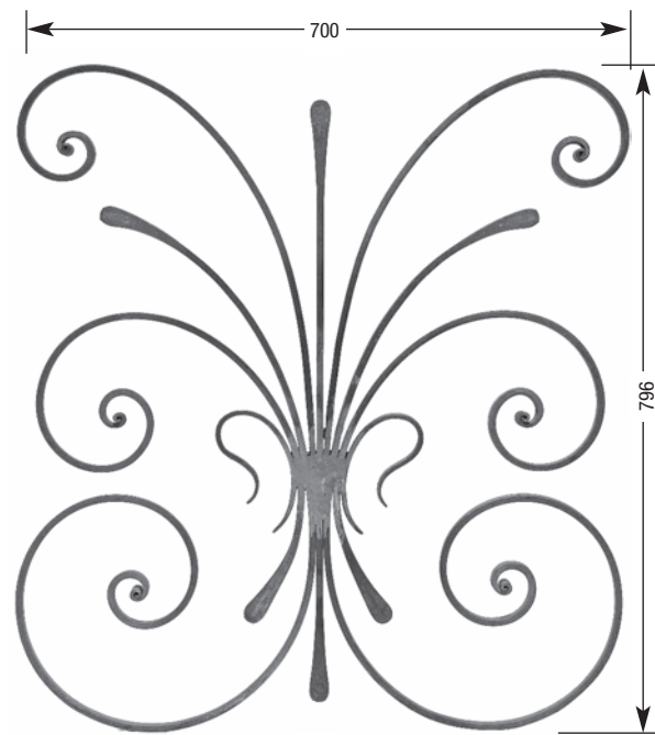
LISSE ART. PANV6 H. 796 - □14 X 8
