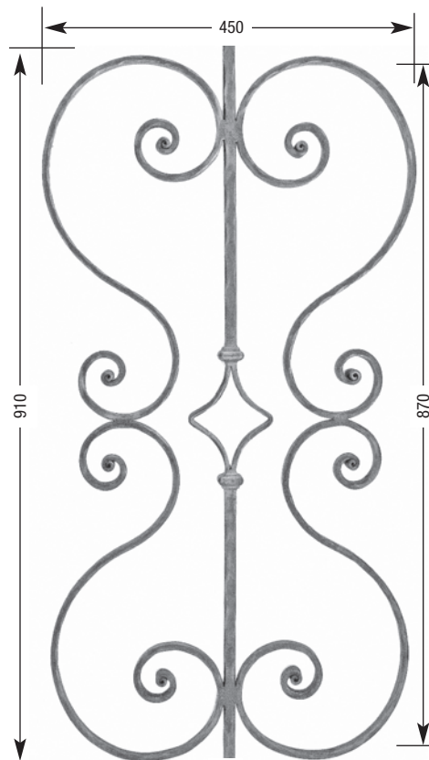
MARTELÉ ART. PAN29-14-910 H. 910 - □14 - Vol. □14x8
