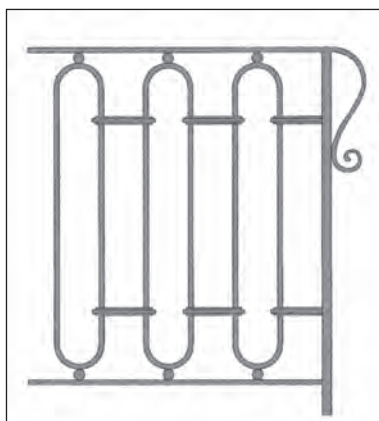
LISSE ART. 64-14-910 H. 910 - □14 ART. 64-14-1200 H. 1200 - □14 ART. 64-14-1500 H. 1500 - □14
