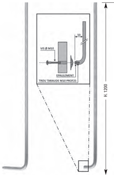
LISSE ART. RL16C1 H. 1200-Ø16 LISSE ART. RL16C2 H. 1200-Ø16 Taraudage M10 LISSE ART. RL14C3 H. 1200-Ø14 2 trous Ø 6,5
