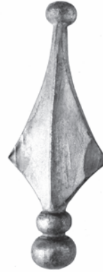
ART. FL4 H. 235 x L 95
